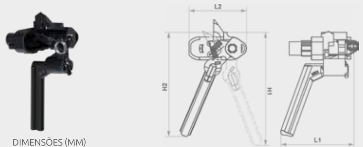
DIMENSÕES (MM)
