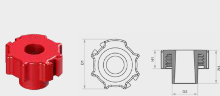
DIMENSÕES (MM)
