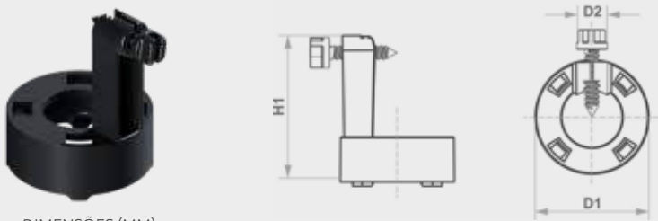
DIMENSÕES (MM)
