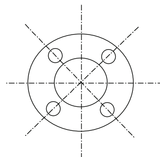
Especificações das flanges TIGRE, furação e parafuso
